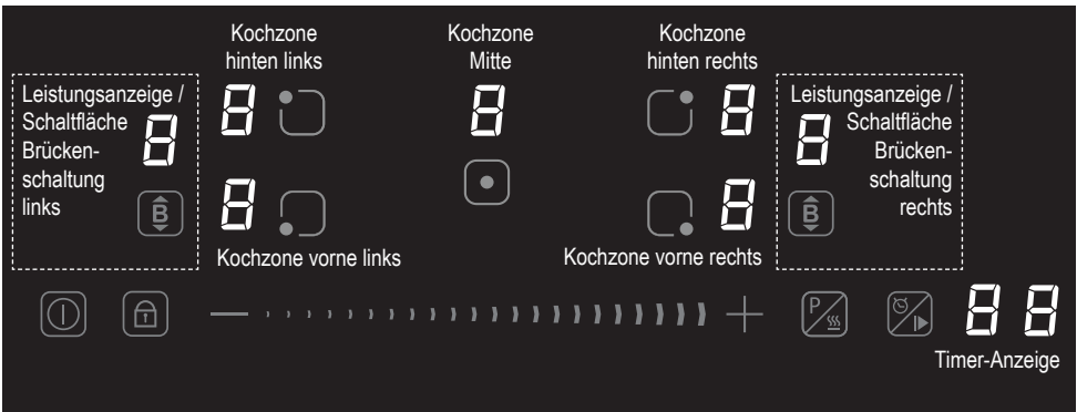
Bedienfeld FLI580
